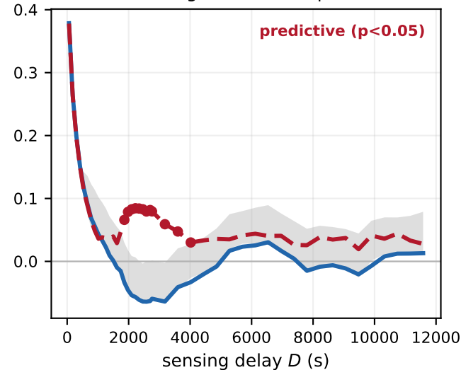
GOES magnetometer · space wx
