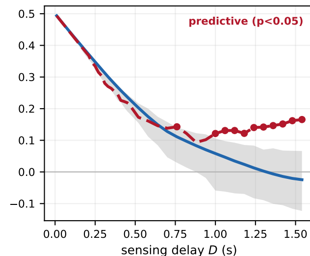
LOCATA VAD · acoustics
