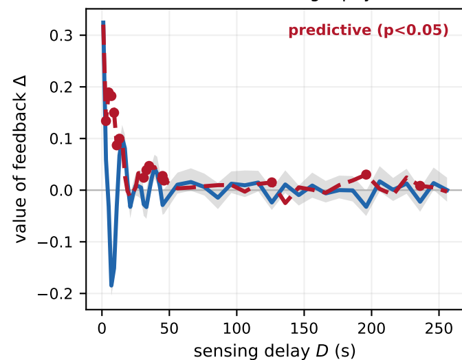
Seismic IU.ANMO · geophysics
