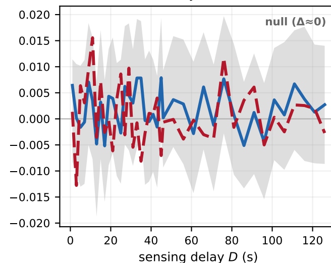
i.i.d. null (synth) · control
