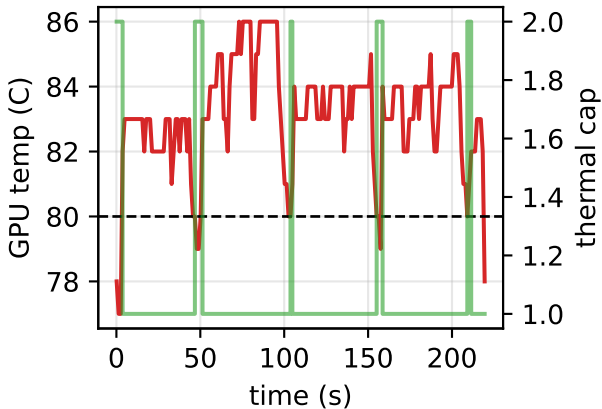
Micro tier: thermal-held burst
