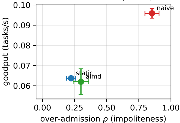
Contended Pareto (poisson)
