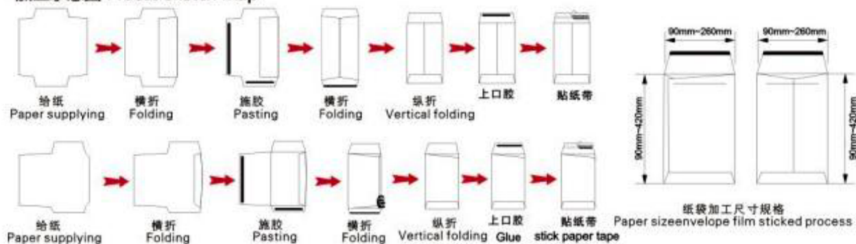
加工示意图 Proess sketch map
