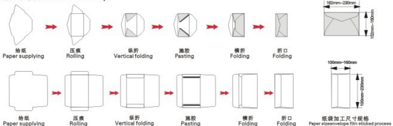
加工示意图 Proess sketch map
