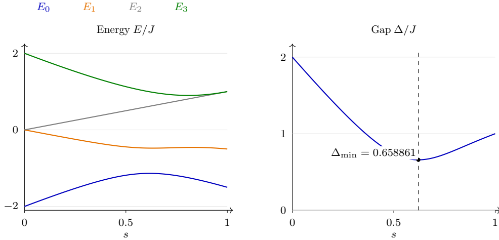
شکل ۶.۲: طیف و گاف محاسبه شده دو اسپین برای h_z = 1/4 ; خط عمودی محل کمینه است. این شکل طرحواره نیست.
