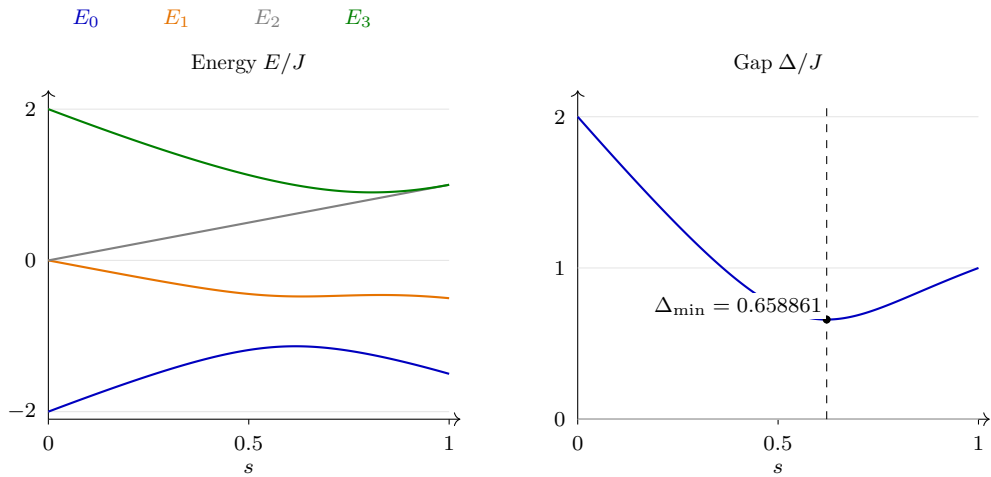
شکل ۷.۲: طیف و گاف محاسبه شده دو اسپین برای h_z = 1/4 ؛ خط عمودی محل کمینه است. این شکل طرحواره نیست.
