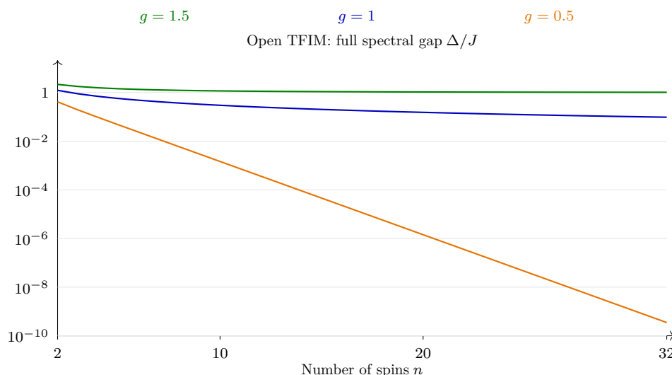
شکل ۹.۲: گاف زنجیره باز از محاسبه مقادیر تکین برای g = 1.5, 1, 0.5 . منحنی فاز مرتب شکافت کم انرژی را نشان می‌دهد، نه گاف حجمی. قدرت محلی J = 1 ثابت است.
