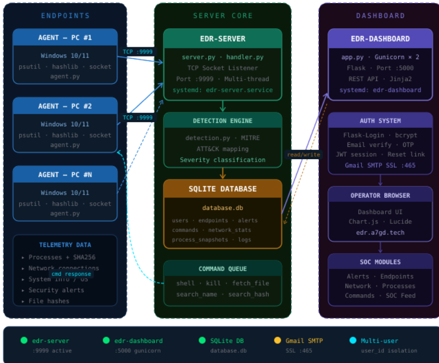
A7_._GD mini EDR PRO - System Architecture - edr.a7gd.tech
