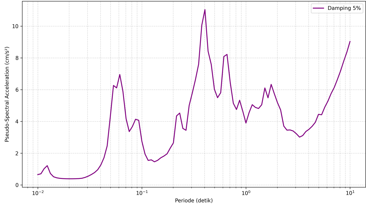
Spektrum Respons (PSA): Stasiun BBJM (HNE)
