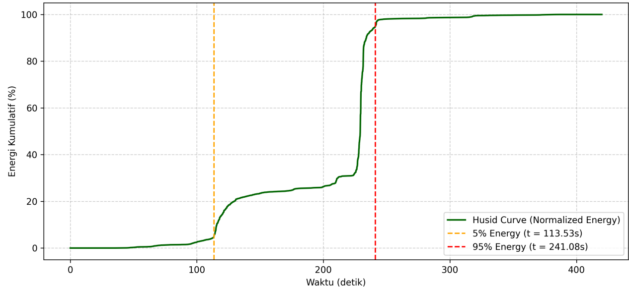
Husid Plot & Durasi Signifikan ( D_{5-95} = 127.55 detik)
