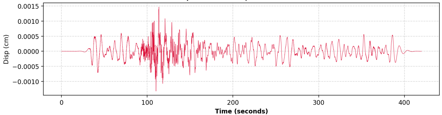
4. Displacement (HNZ | PGD: 0.001466 cm)
