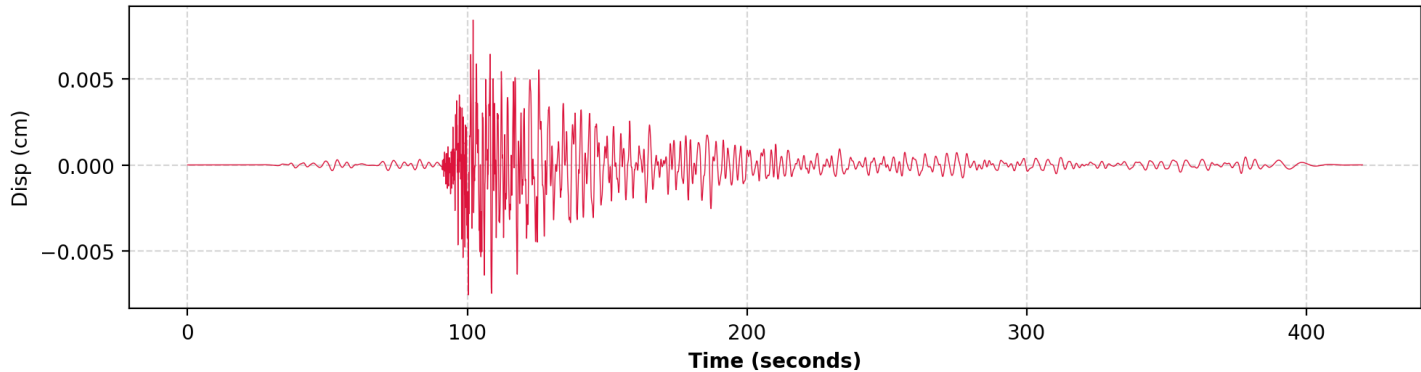
4. Displacement (HNZ | PGD: 0.008407 cm)
