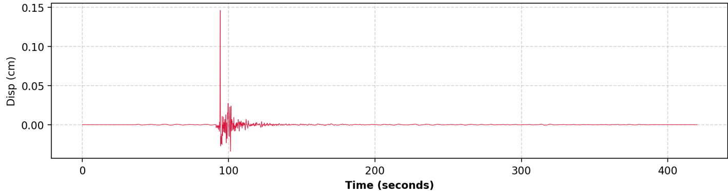
4. Displacement (HNE | PGD: 0.146305 cm)
