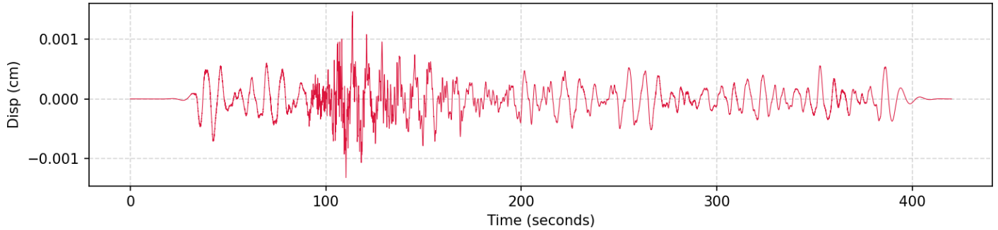
4. Displacement (HNZ | PGD: 0.001466 cm)
