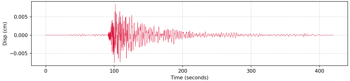
4. Displacement (HNZ | PGD: 0.008407 cm)
