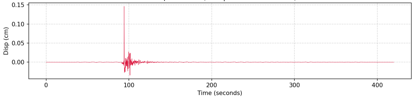
4. Displacement (HNE | PGD: 0.146305 cm)
