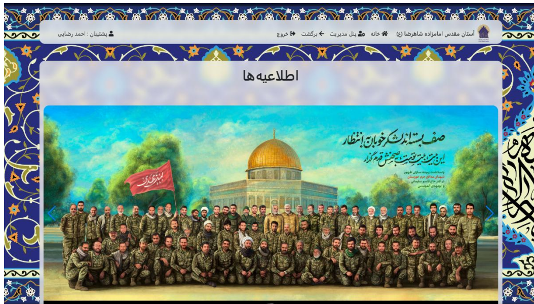
شکل ۴-۲ صفحه خانه
