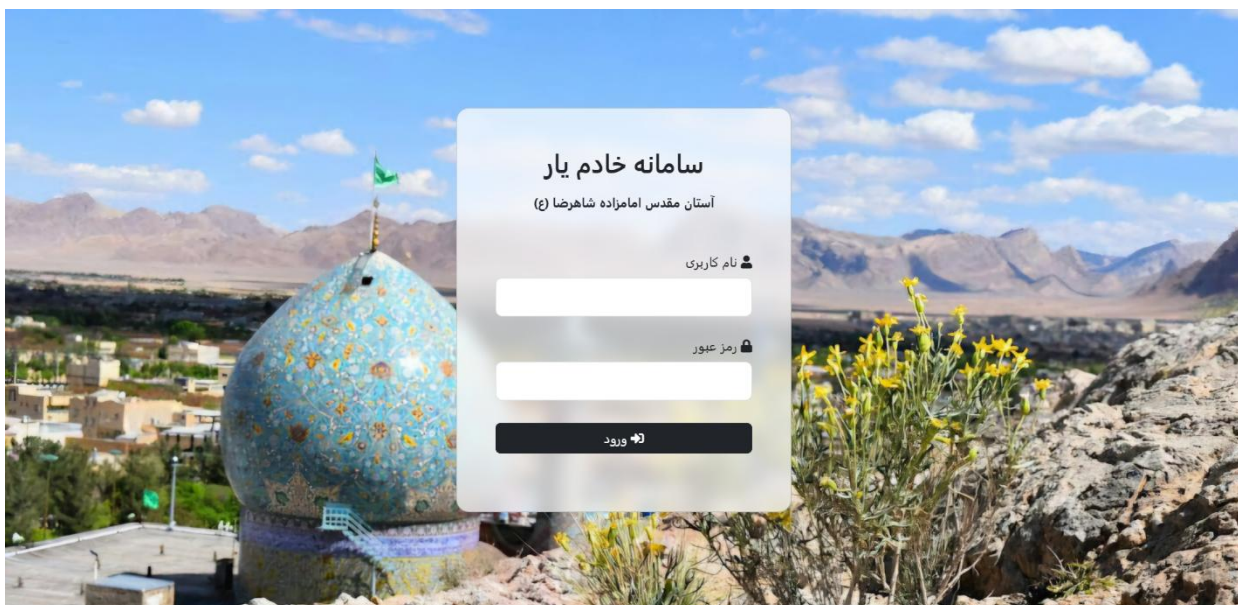
شکل ۴-۱- صفحه ورود
