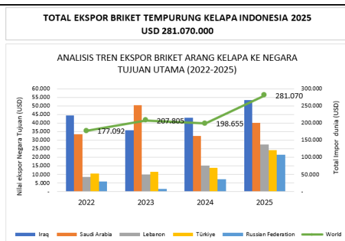
Gambar 7 Tren Ekspor Briket Arang Tempurung Kelapa Indonesia Ke Negara Tujuan Utama (2022-2025)
