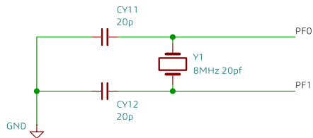
8MHZ OSCILLATOR
