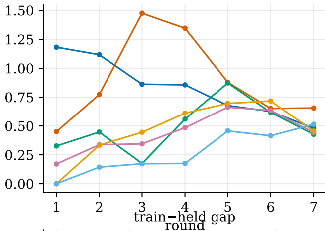
LoRA drift
