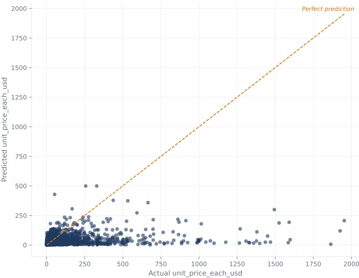
Predicted vs actual · holdout n = 3800
