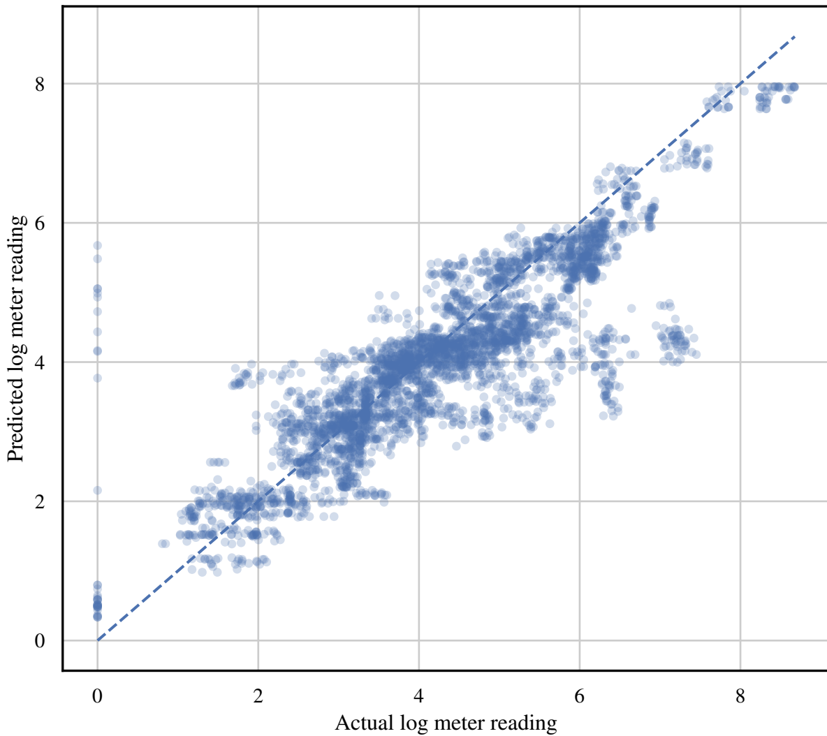
Predicted vs Actual: CatBoost
