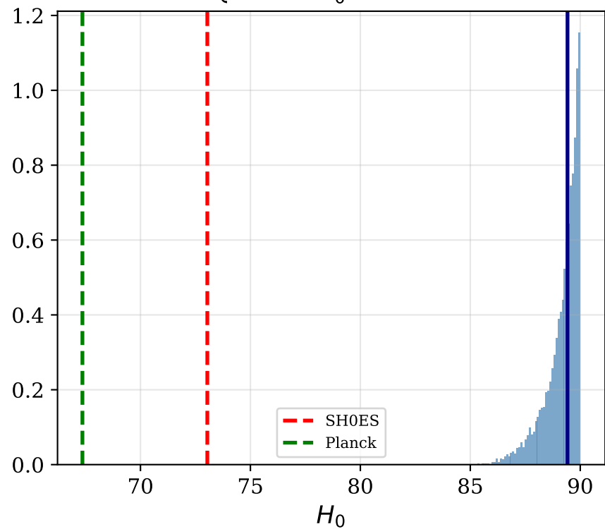
EQST-GP H_0 Posterior
