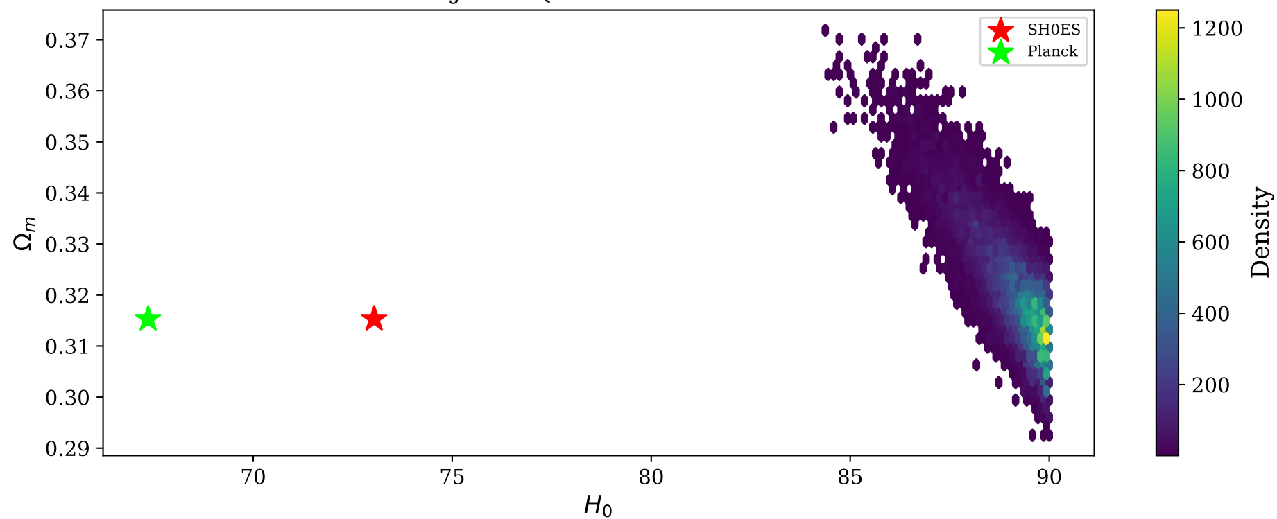
Joint EQST-GP Posterior
