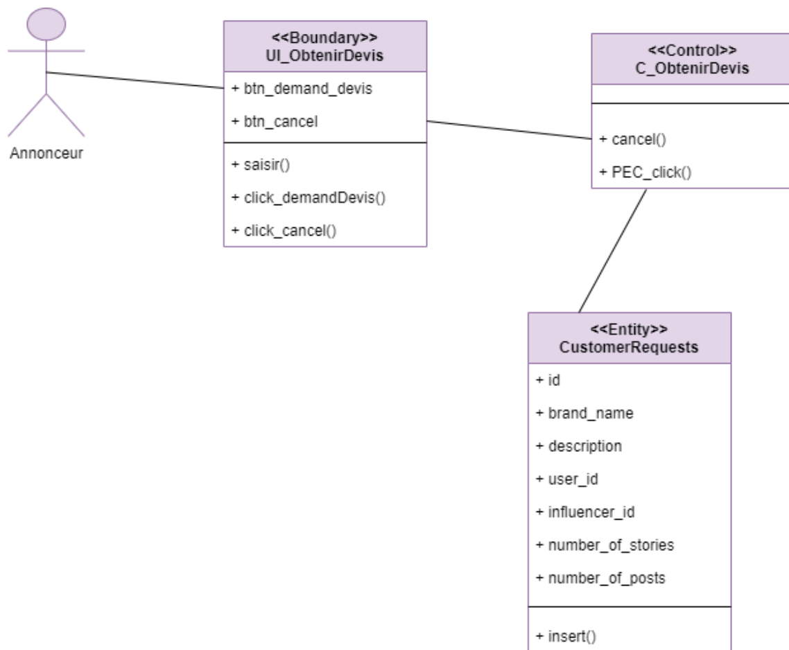
FIGURE 4.14 – Diagramme de classe du cas d'utilisation «Obtenir devis»
