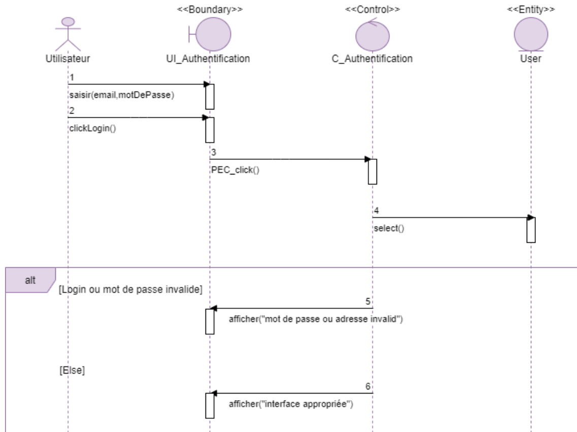
FIGURE 3.6 – Diagramme de séquence du cas d'utilisation «S'authentifier»
