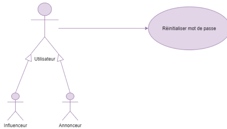
FIGURE 3.4 – Raffinement de cas d'utilisation «Réinitialiser mot de passe»
