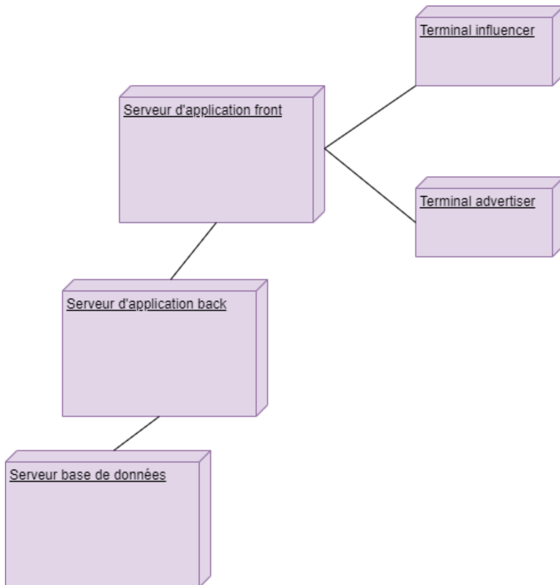
FIGURE 3.13 – Diagramme de déploiement
