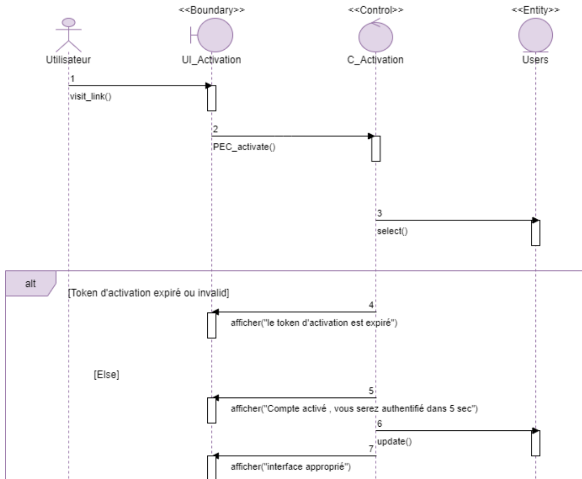
FIGURE 3.10 – Diagramme de séquence de sous cas d'utilisation «Activer compte»
