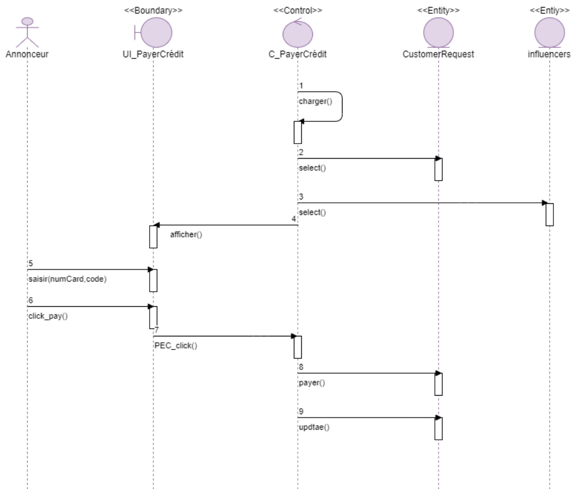
FIGURE 4.19 – Diagramme de séquence du cas d'utilisation «Payer crédit»
