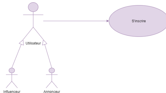
FIGURE 3.2 – Raffinement de cas d'utilisation «S'inscrire»
