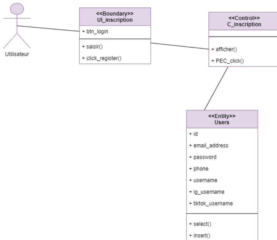
FIGURE 3.7 – Diagramme de classe du cas d'utilisation«S'inscrire»
