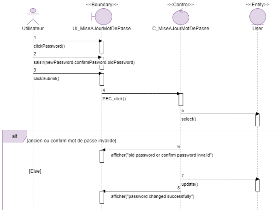
FIGURE 4.9 – Diagramme de séquence du cas d'utilisation «Mettre à jour mot de passe»
