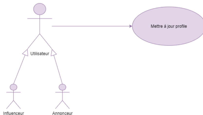
FIGURE 4.2 – Raffinement de cas d'utilisation «Mettre à jour profile»
