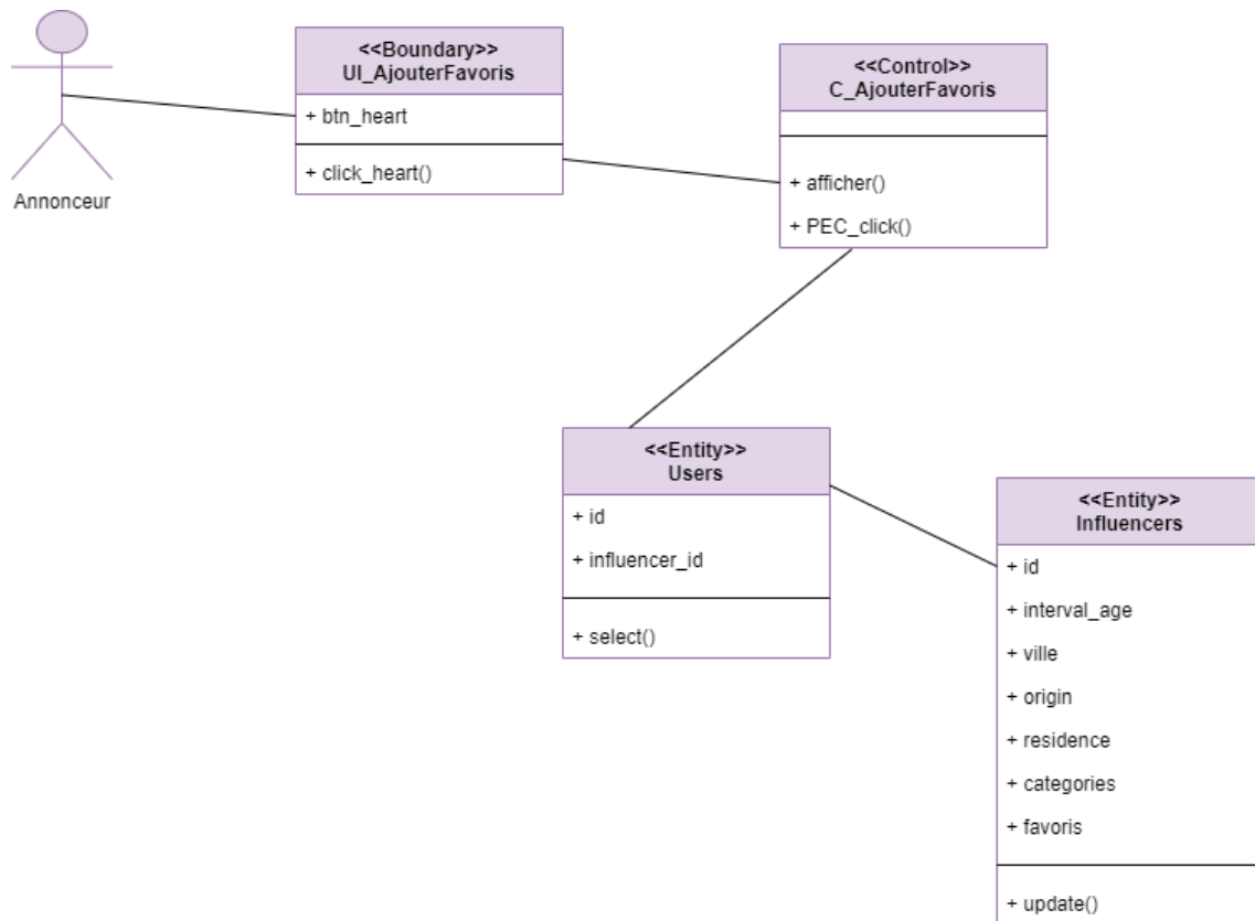
FIGURE 4.16 – Diagramme de classe du cas d'utilisation «Ajouter influenceur favoris»
