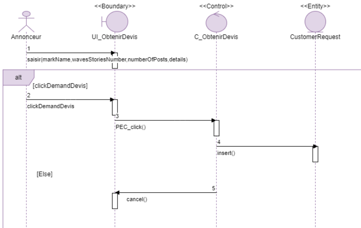
FIGURE 4.15 – Diagramme de séquence du cas d'utilisation «Obtenir devis»
