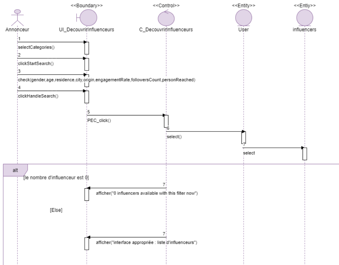
FIGURE 4.13 – Diagramme de sequence du cas d'utilisation «Découvrir influenceurs»
