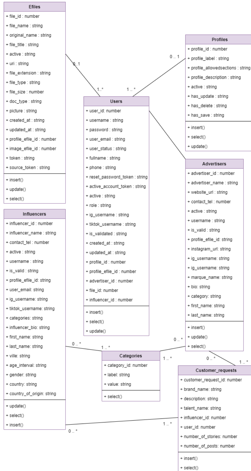
FIGURE 2.3 – Diagramme de classe globale
