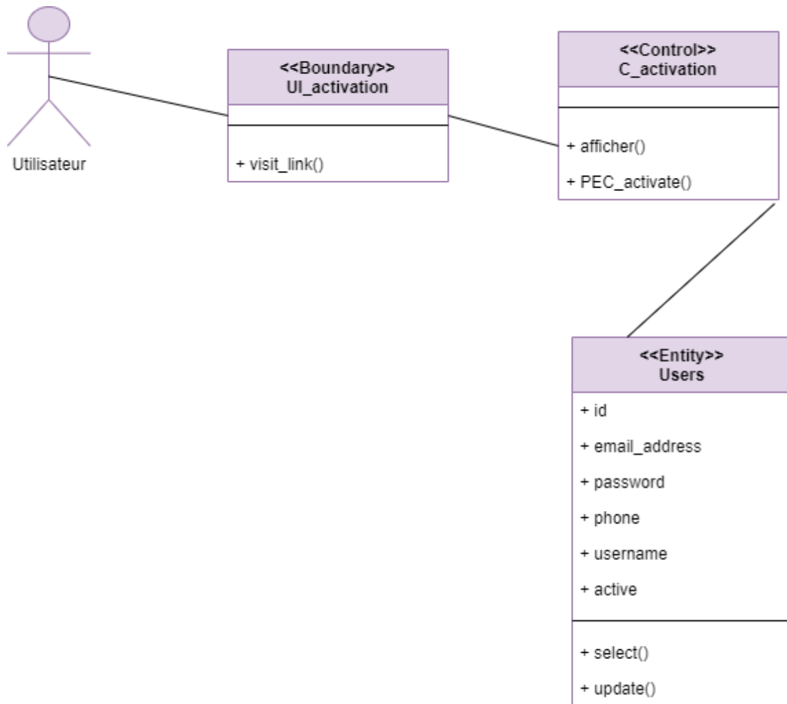
FIGURE 3.9 – Diagramme de classe de sous cas d'utilisation «Activer compte»
