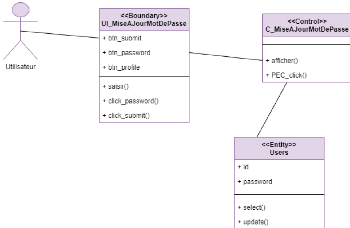
FIGURE 4.8 – Diagramme de classe du cas d'utilisation «Mettre à jour mot de passe»
