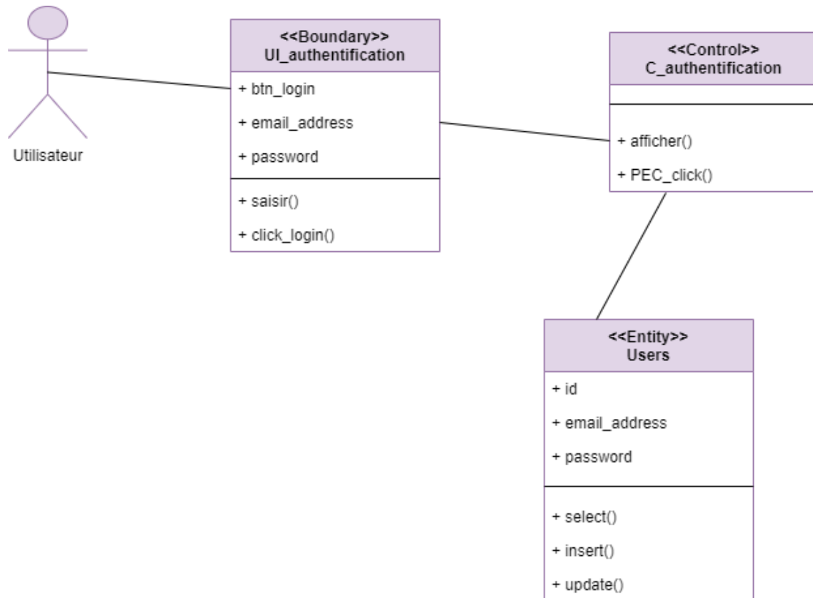
FIGURE 3.5 – Diagramme de classe du cas d'utilisation «S'authentifier»
