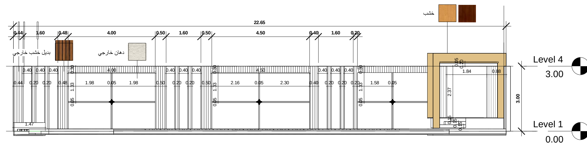
مخطط الواجهه الغربيه
