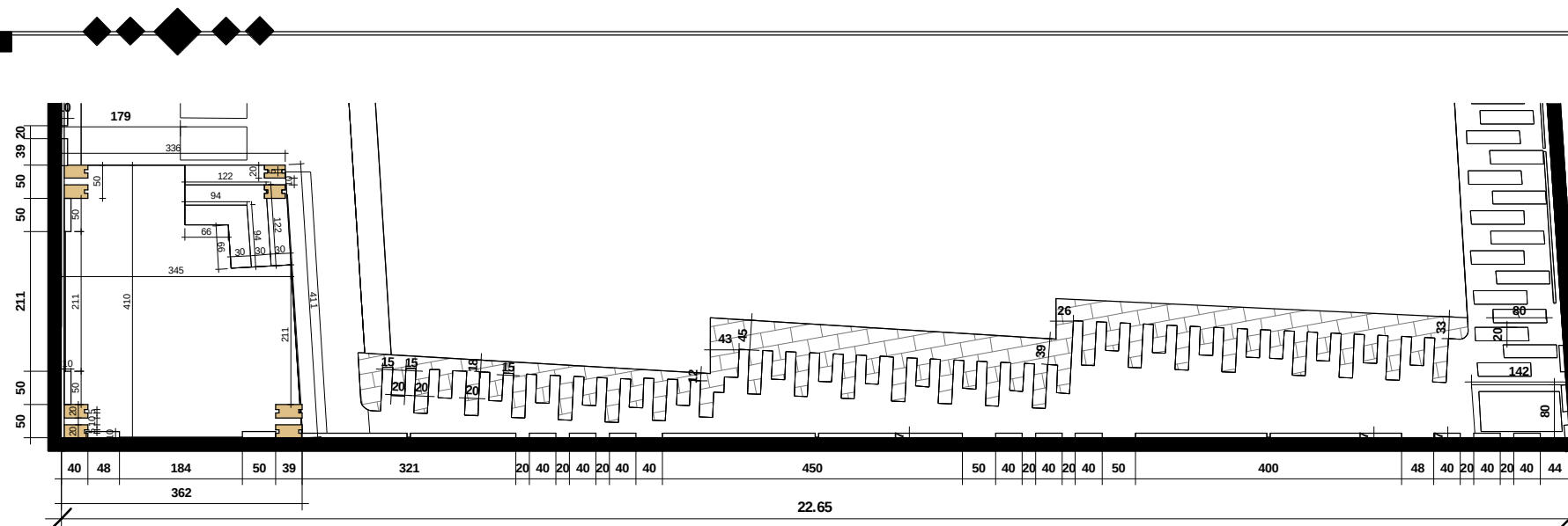
مسقط الواجهه الغربيه
