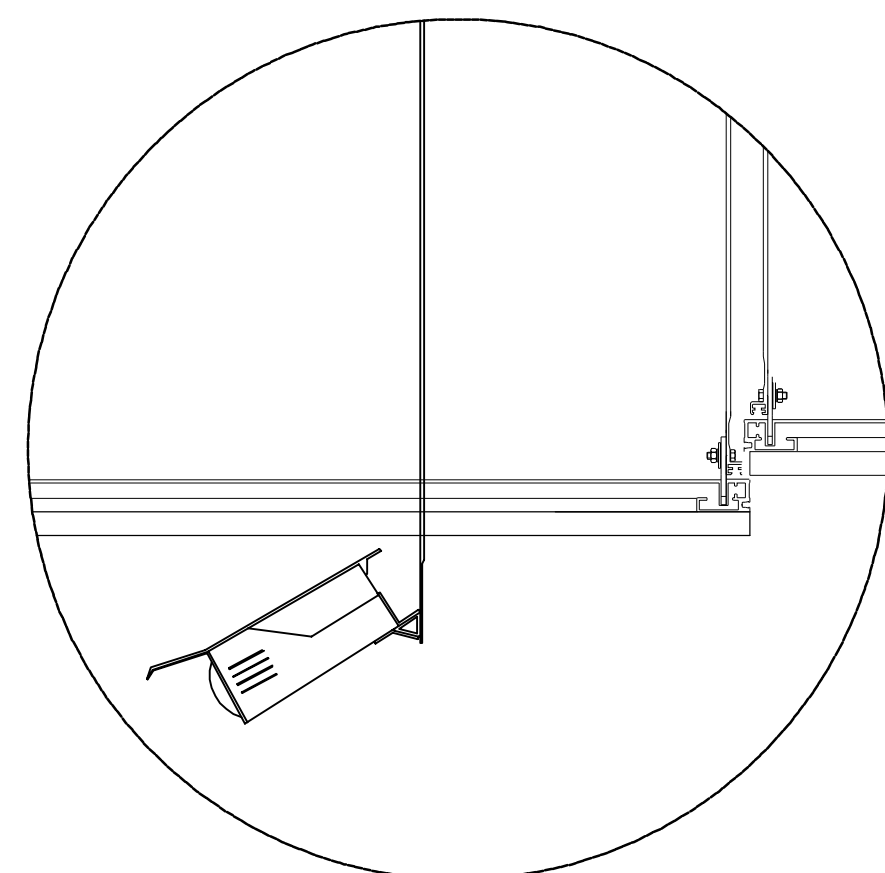
تفصيلة إضاءة سقف المسرع مقياس رسم 10/1
