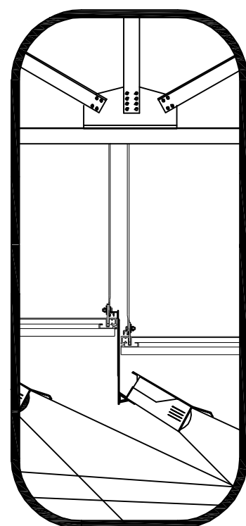
تفصيلة الإنارة المتحركة في خلية المسرع مقياس رسم 10/1
