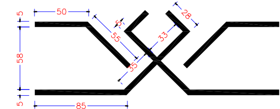
تفصيلة نقطة الواجبه مقياس رسم 25/1
