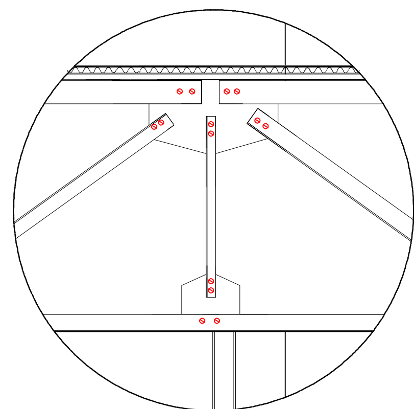
تفصيلة السقف الانشائي مقياس رسم 10/1
