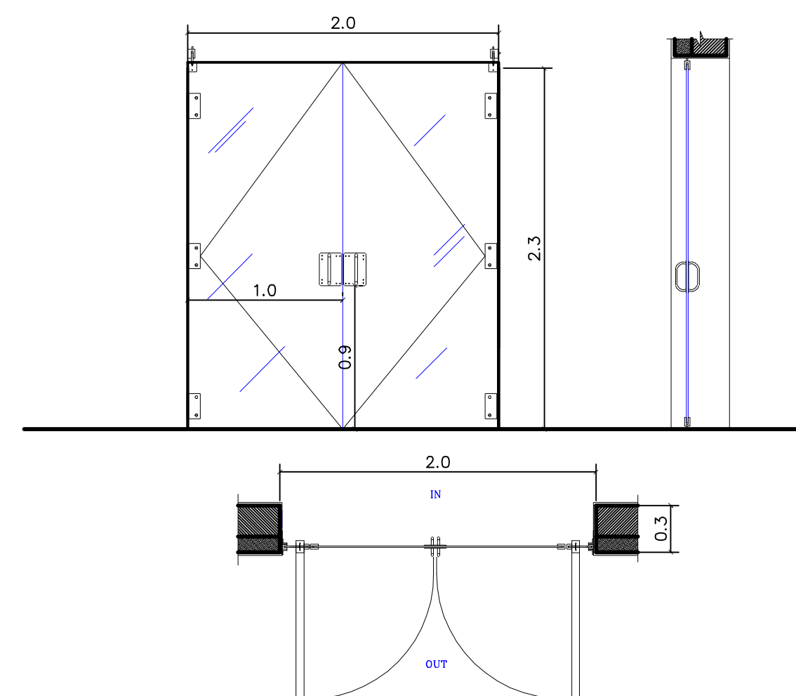
تفصيلة باب مقياس رسم 25/1
