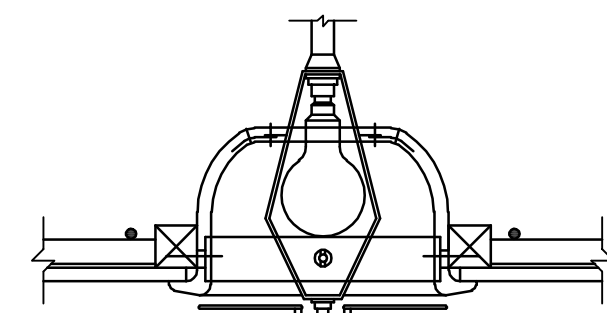
تفصيلة توضع الإضاءة في سقف المسرع مقياس رسم 10/1
