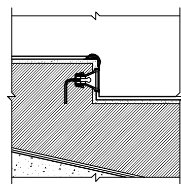
تفصيلة توضع الإضاءة في درج المسرع مقياس رسم 10/1
