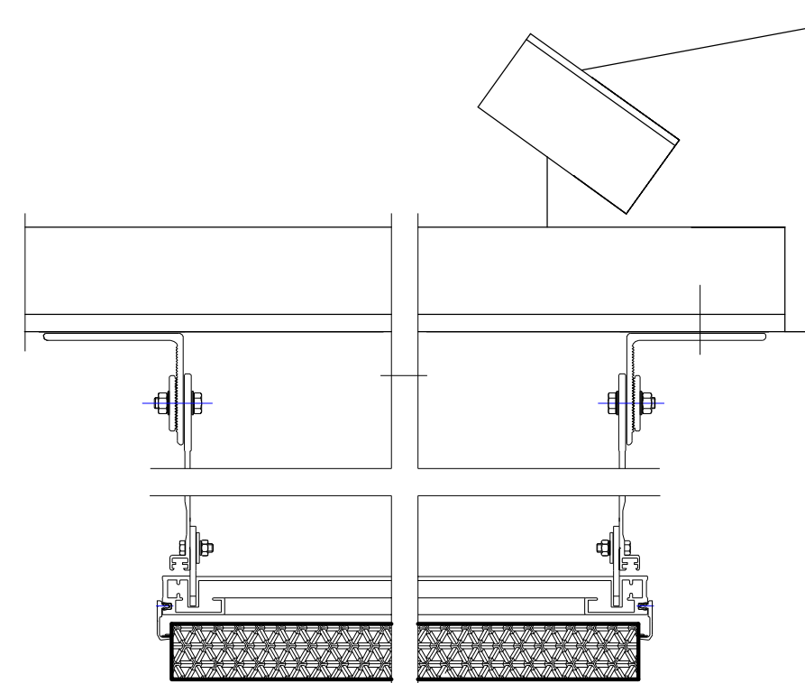
تفصيلة توضع السقف المستعار مقياس رسم 10/1
