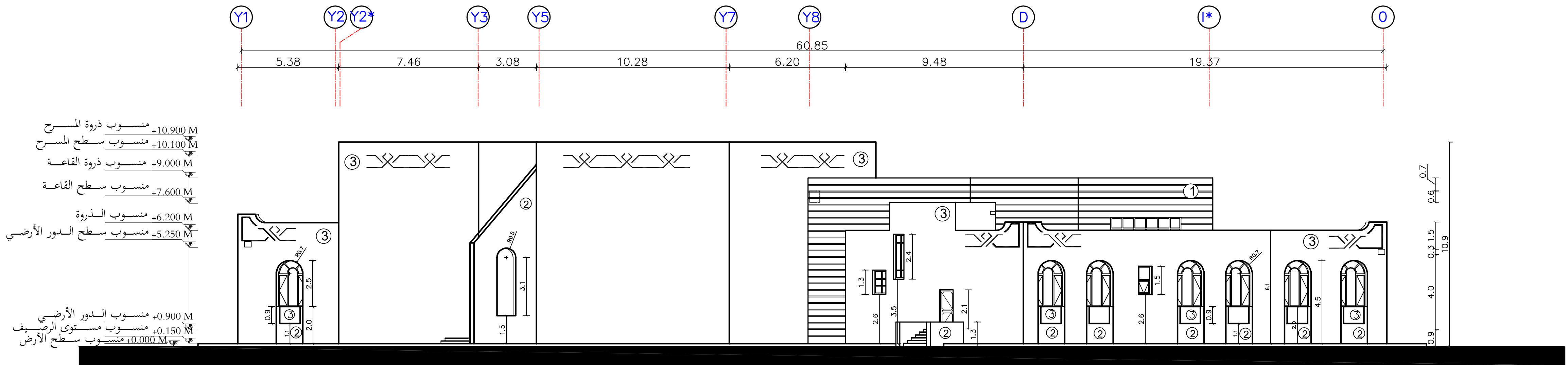
الواجهة الغربية مقياس رسم 100/1
