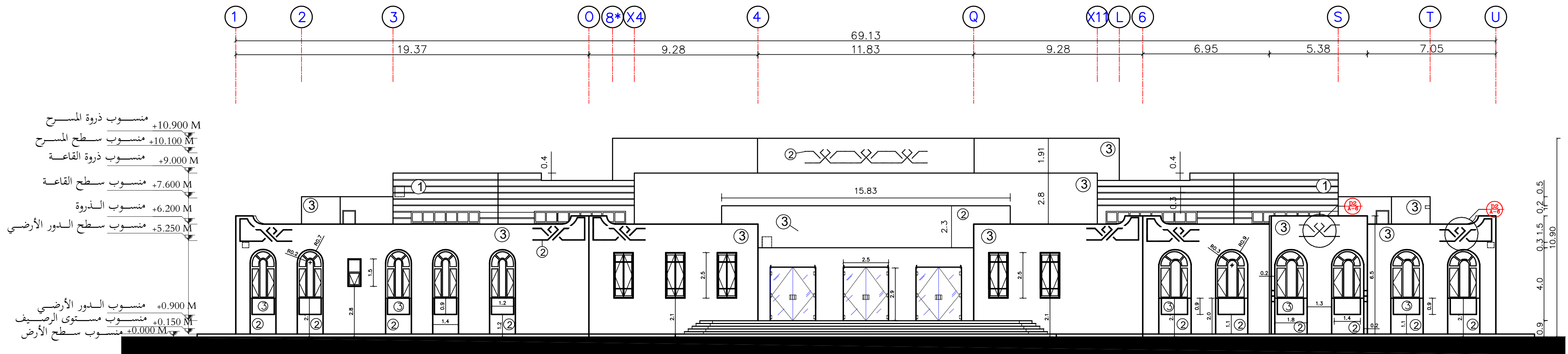
الواجهة الجنوبية مقياس رسم 100/1
