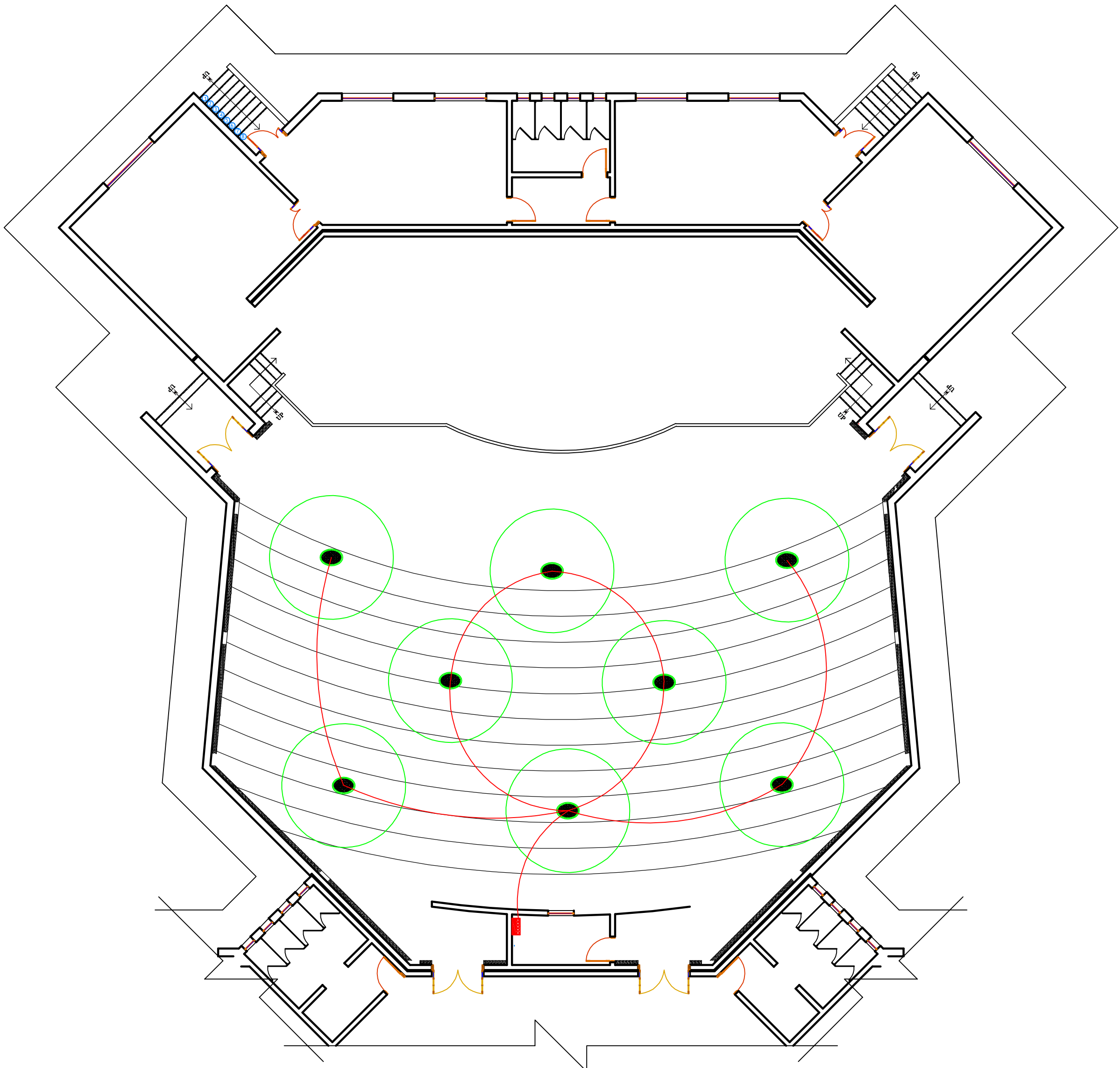
شعريانية صوتية المسرح مقياس رسم 100/1
