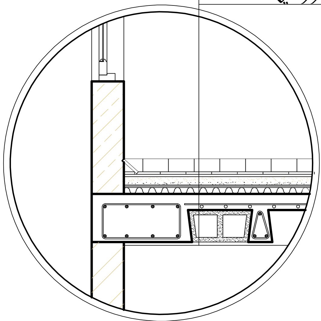
التفصيلة رقم 10 مقياس رسم 10/1
