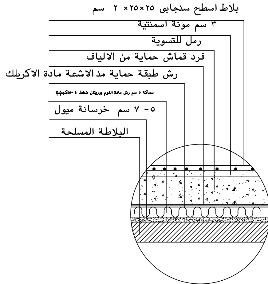
تفصيلة بلاطة السقف العلوى ( ٣ )
