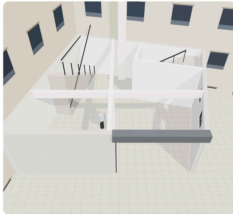
الدور الأول ≈ ٨٩ م²: باب رول ٤.٥ م على شارع ١٢، وسلم داخلي للدور الثاني على حيطه الجار.
