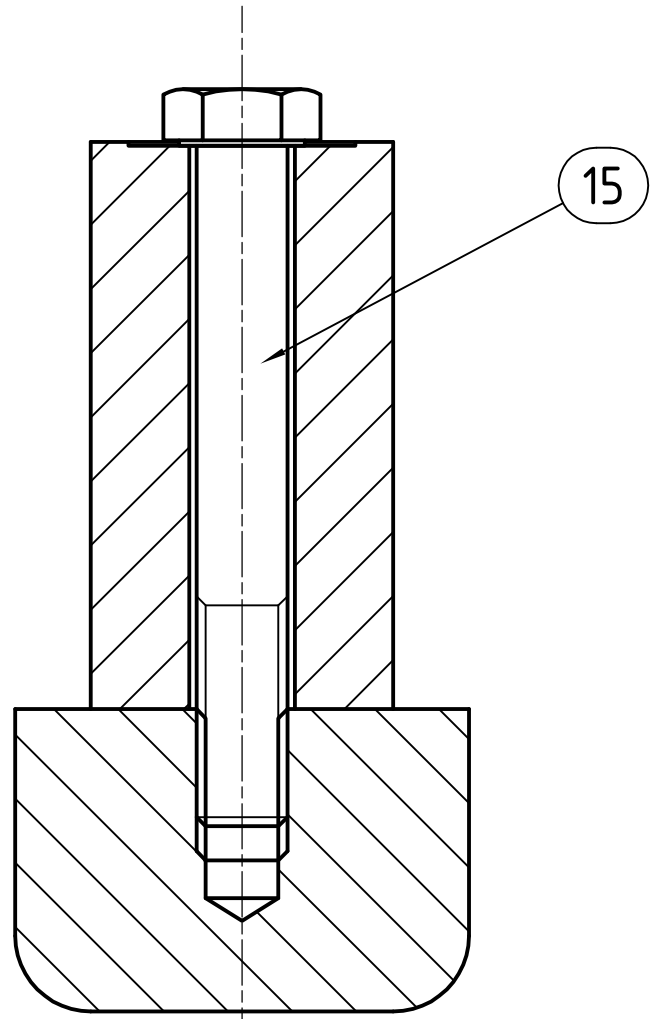
B-B SCALE 1:1
