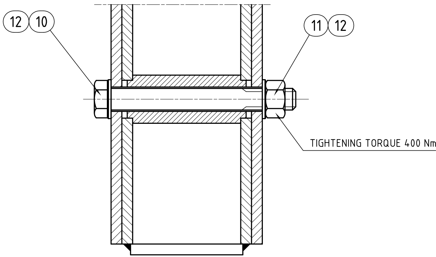
C-C SCALE 1:2
