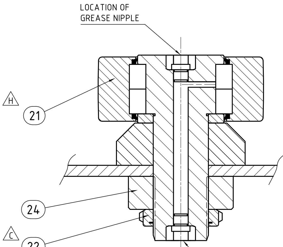
D-D SCALE 1:1
