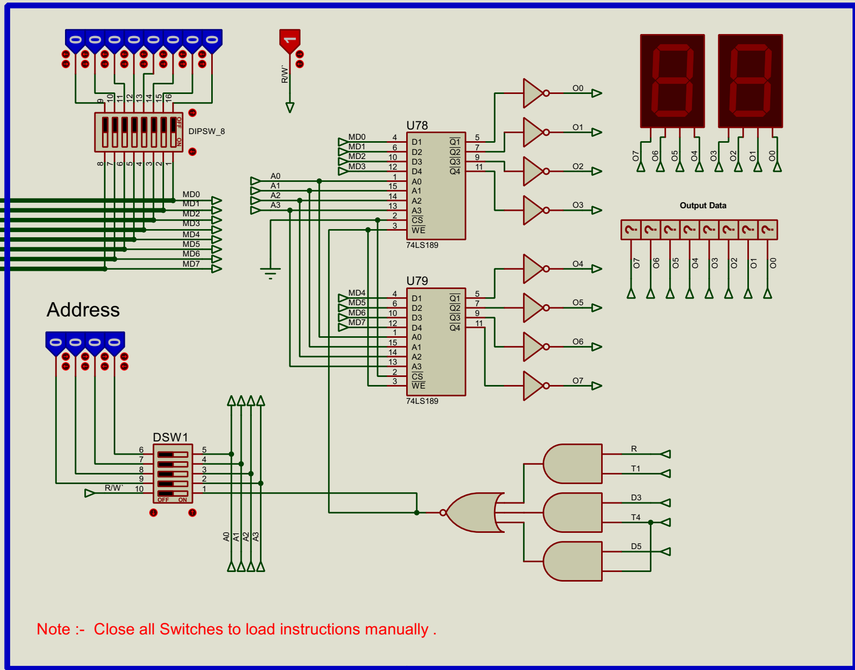
RAM_16X8
