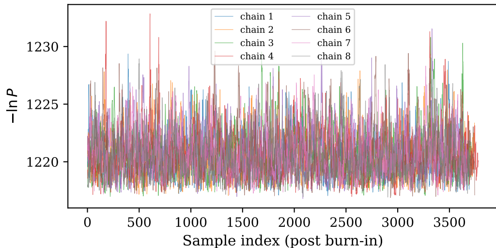
-\ln P trace per chain
