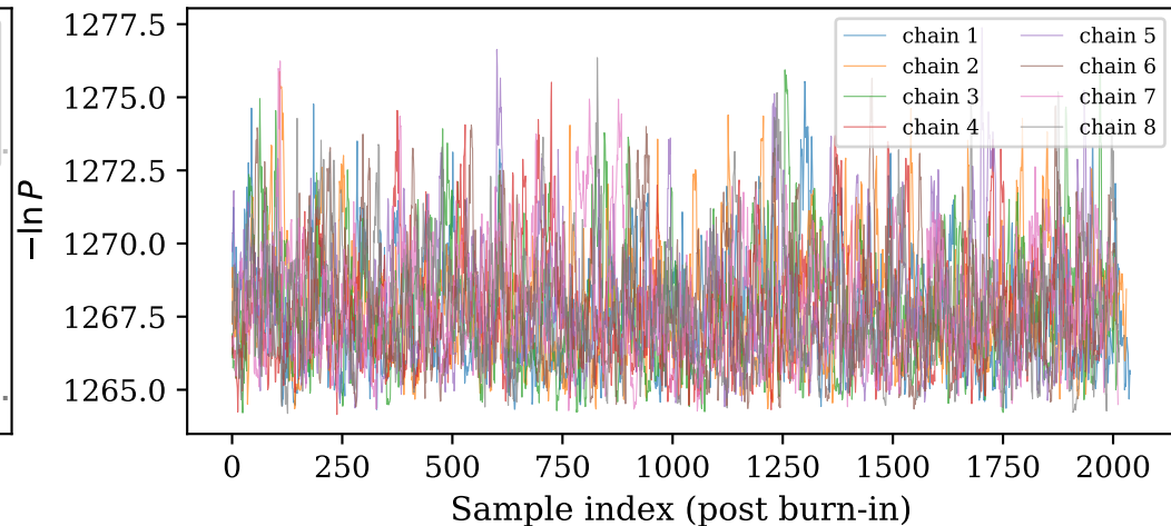
-\ln P trace per chain
