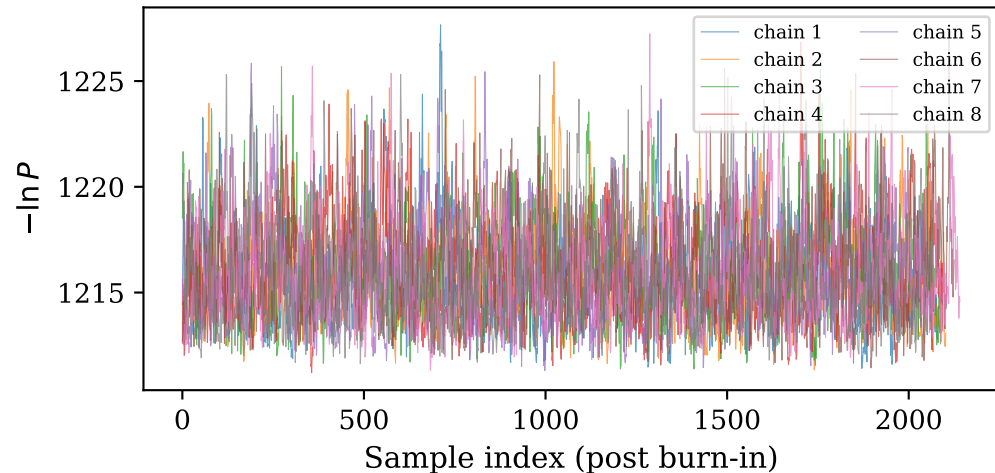
-\ln P trace per chain
