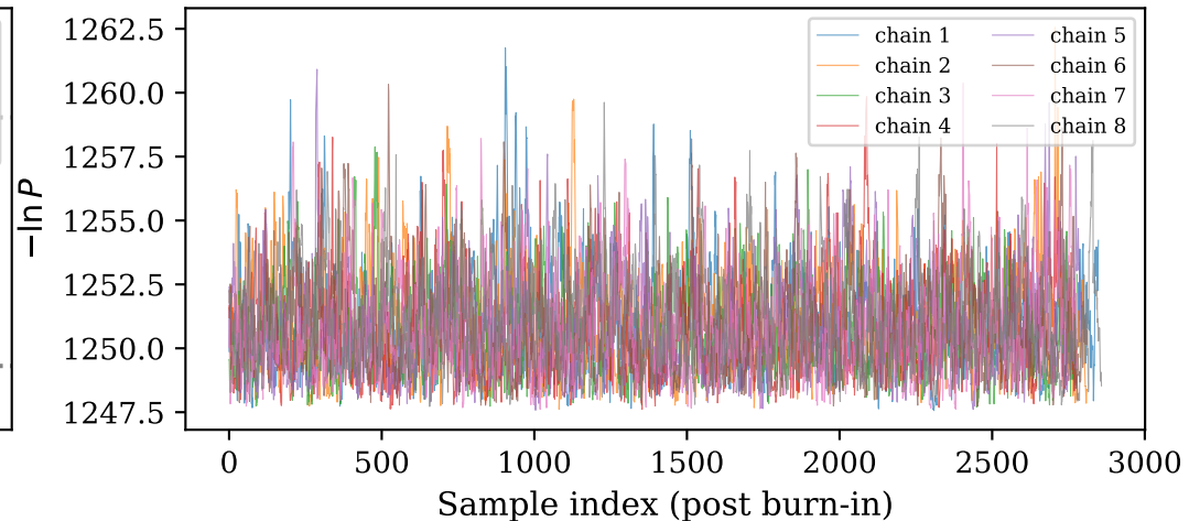
-\ln P trace per chain
