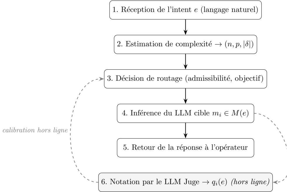
FIGURE 4.2 – Flux de traitement d’un intent par InferRouter-LLM. Les étapes 1 à 5 forment le chemin critique et correspondent aux termes de la décomposition de latence (§3.3.7) ; la latence de transport réseau y est absorbée par la co-localisation du routeur en bordure. La notation par le juge (étape 6, en gris) n’y figure pas : elle s’exécute hors ligne et ne retarde pas la réponse à l’opérateur.
