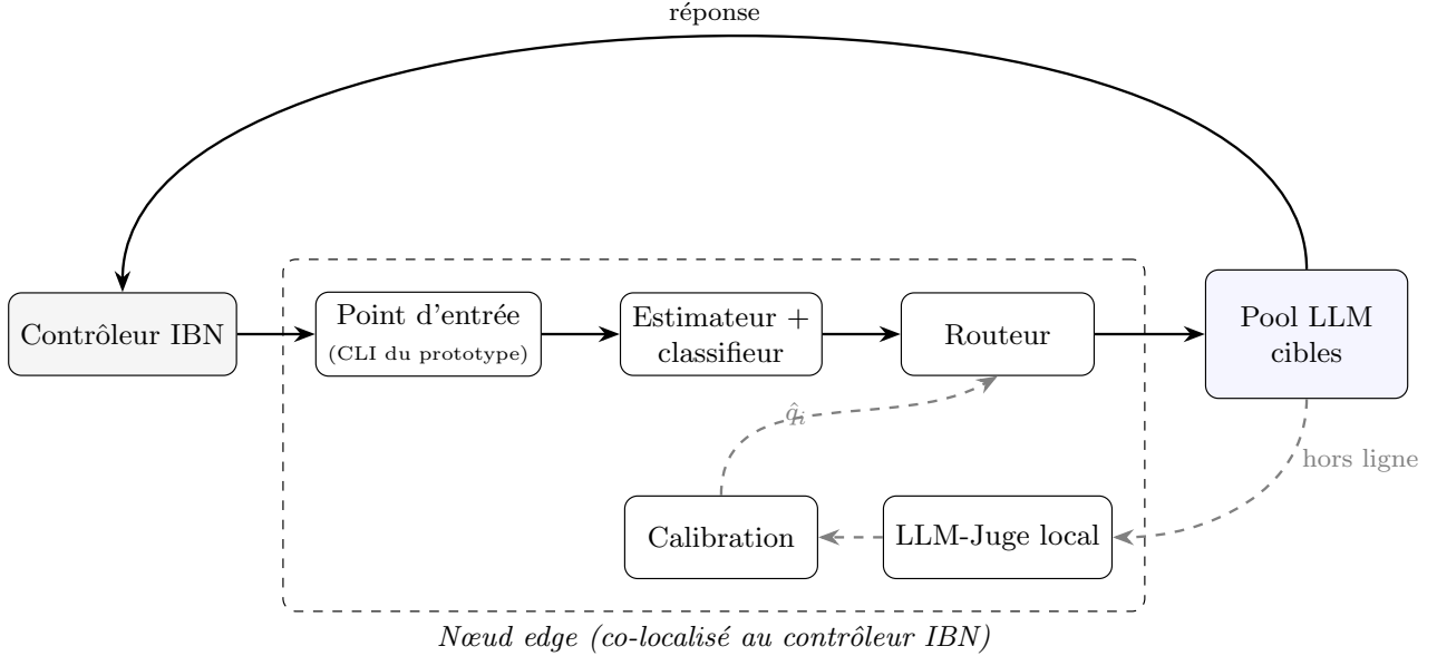
FIGURE 4.1 – Architecture système d’InferRouter-LLM. Le chemin critique (traits pleins) enchaîne estimation, routage et inférence du modèle sélectionné R^*(e) , appelé en cloud. La co-localisation du routeur avec le contrôleur réseau rend le transport intra-cluster négligeable devant l’inférence cloud, de l’ordre de la dizaine de secondes (Table 4.1). Les traits pointillés ne décrivent pas une boucle au runtime : le LLM-Juge note les réponses hors chemin critique, et ses mesures alimentent entre deux campagnes la table de qualité attendue \hat{q}_i que le routeur consulte (§4.7).
