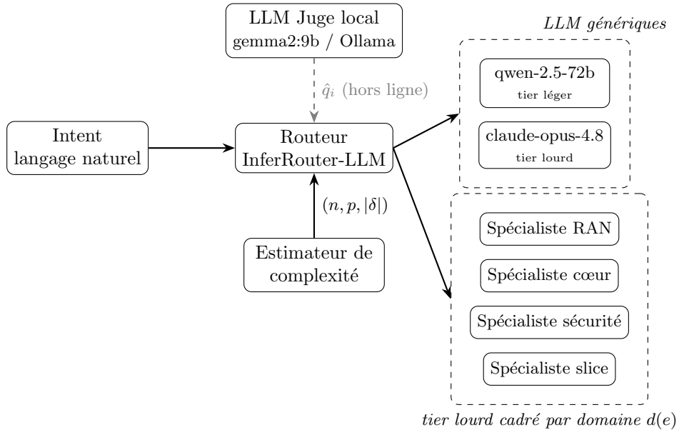
FIGURE 4.3 – Architecture du pool de LLM cibles d’InferRouter-LLM. Le routeur sélectionne entre deux génériques, un tier léger et un tier lourd, et quatre candidats où le tier lourd est cadré sur un domaine fonctionnel (RAN, cœur, sécurité, slice) ; ce cadrage n’implique aucun comportement agentique (§4.5.1). L’estimateur fournit au routeur les attributs (n(e), p(e), |\delta(e)|) sur le chemin critique. Le LLM Juge, lui, n’intervient pas dans la décision : ses mesures a posteriori q_i(e) alimentent hors ligne la table de qualité attendue \hat{q}_i que le routeur consulte (§4.7).
