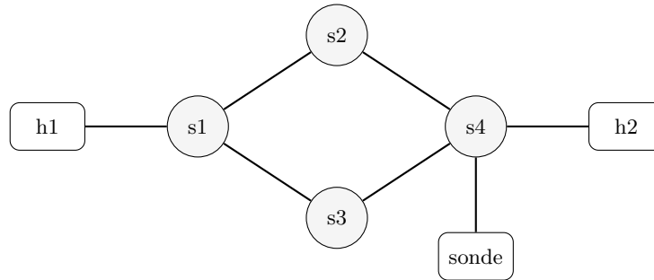
FIGURE 5.2 – Topologie du banc émulé (Mininet pilotant des commutateurs Open vSwitch). Le losange à quatre commutateurs ( s1–s4 ) offre deux chemins entre l’hôte source h1 et l’hôte destination h2 , ce qui rend le reroutage observable dans le plan de données. L’hôte sonde reçoit les flux dupliqués. Les commutateurs opèrent en mode secure : le banc installe lui-même l’acheminement de base, sans apprentissage d’adresses.
