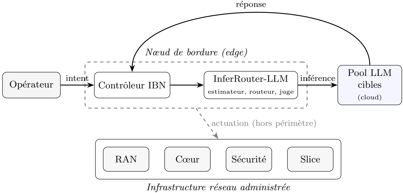
FIGURE 4.2 – Déploiement d’InferRouter-LLM en bordure de réseau. L’opérateur soumet un intent au contrôleur IBN, co-localisé avec InferRouter-LLM sur un nœud de bordure. Le routeur sélectionne un modèle du pool appelé en cloud, dont la réponse revient à l’opérateur. L’actuation sur l’infrastructure administrée (RAN, cœur, sécurité, slice) reste hors périmètre (trait pointillé) : elle relève des phases aval de la boucle IBN (§4.3).
