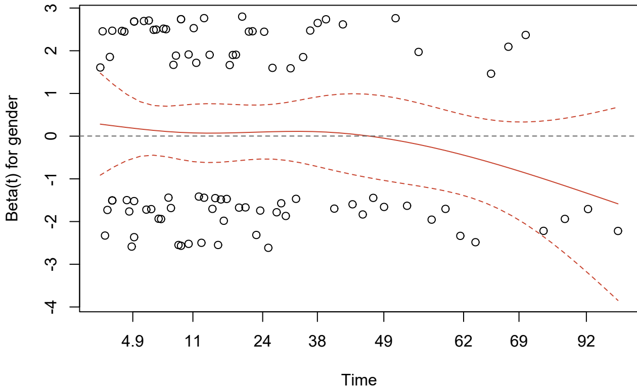
ROCK2 — multivariable: gender (p = 0.227)
