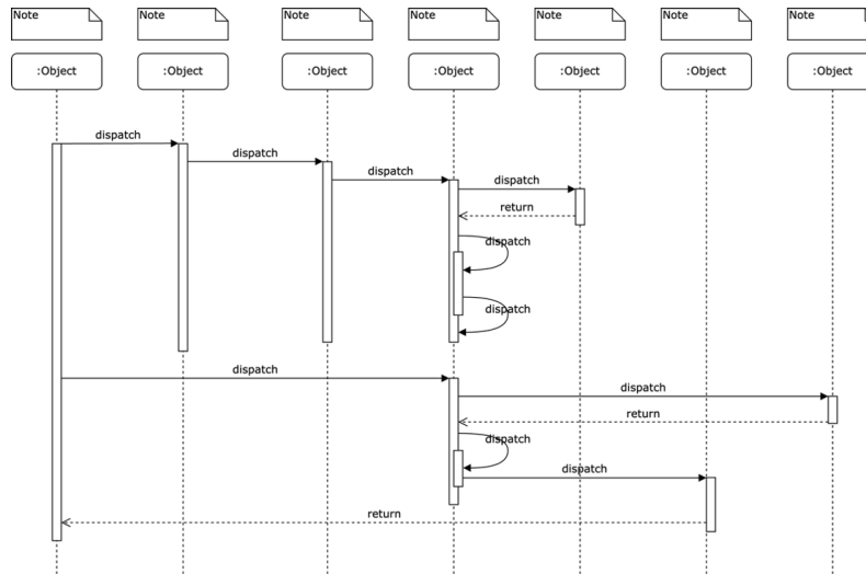
Gambar III.1 Diagram Interaksi Antarobjek pada Sistem ABC
