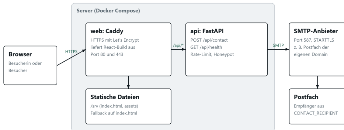
Abbildung 10: Systemarchitektur beim Betrieb mit eigenem Server Quelle: eigene Darstellung
