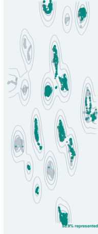
source-label scope
