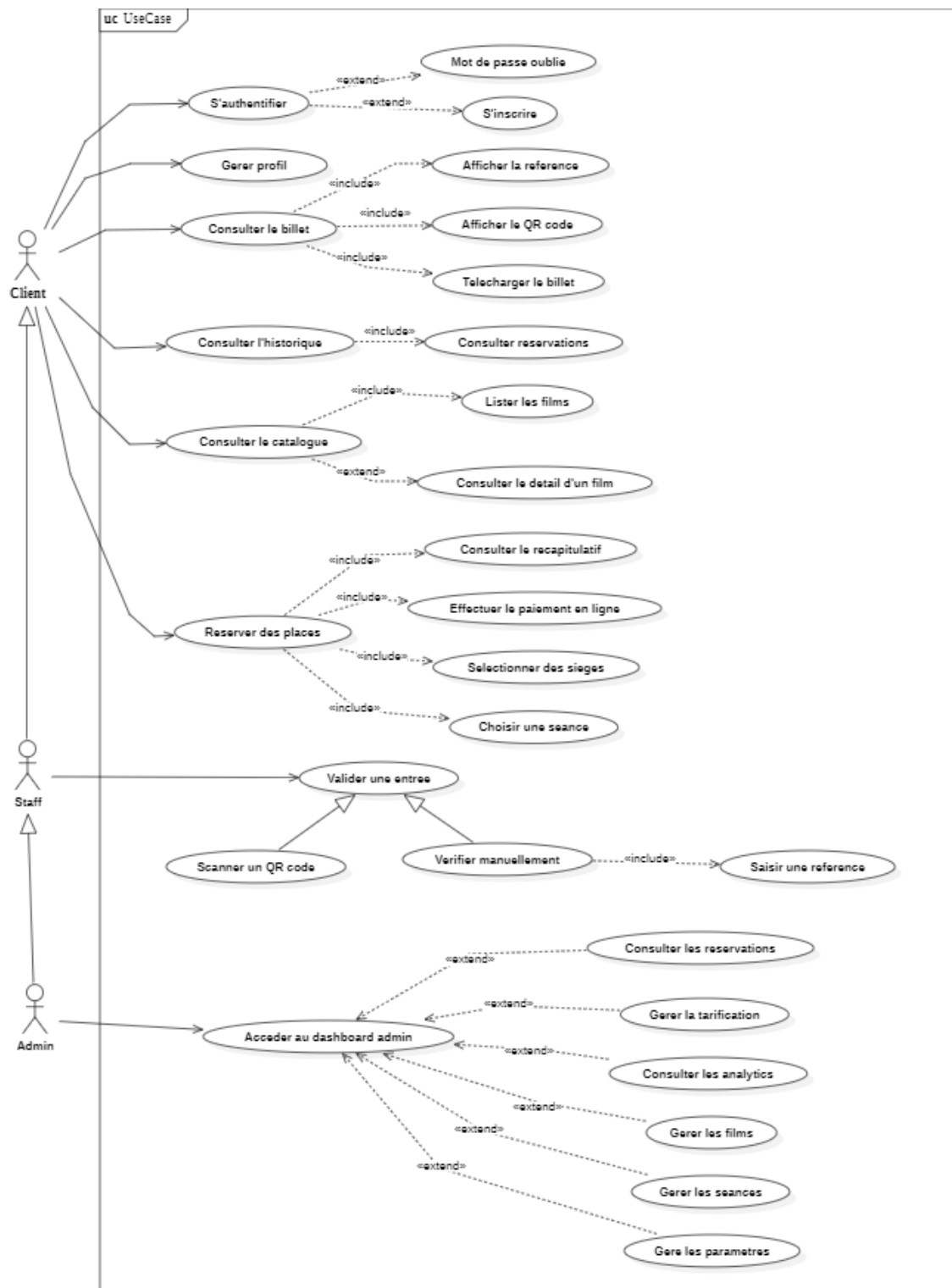
FIGURE 3.1 – Diagramme de cas d'utilisation de CinePass
