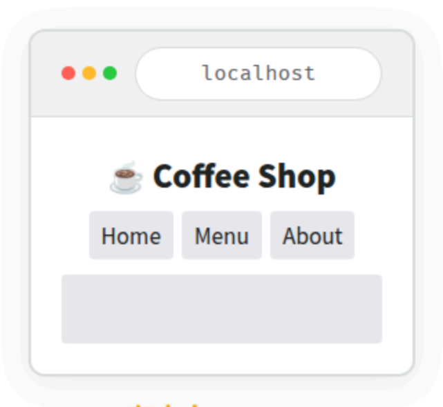
有方向 Prompt
