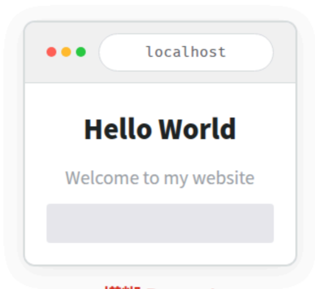
模糊 Prompt
