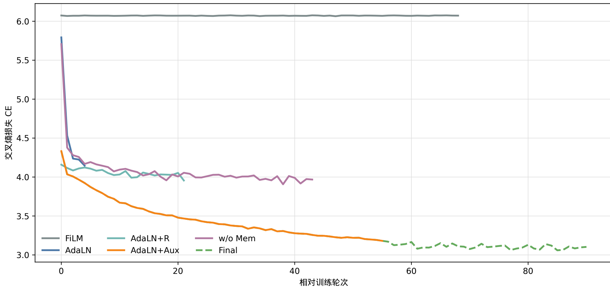
六组消融实验 CE 损失曲线
