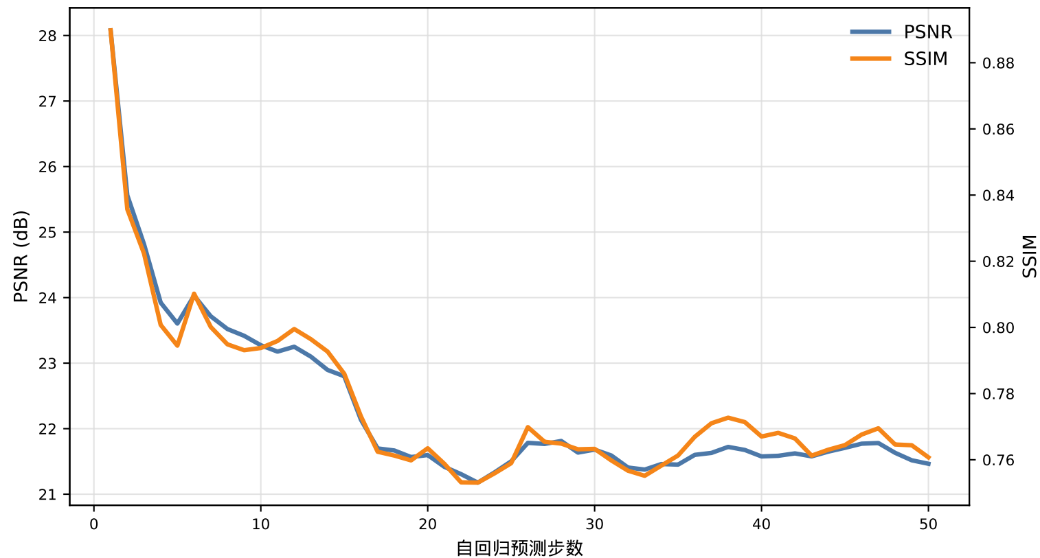
长程自回归质量变化曲线
