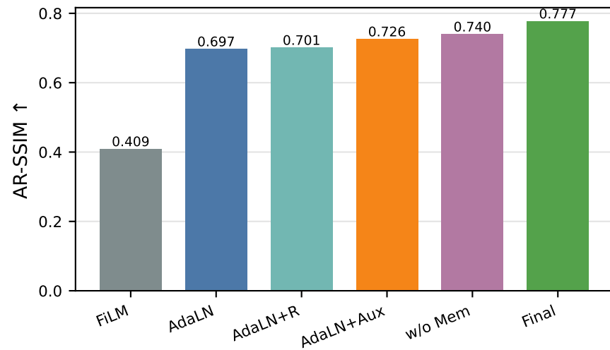
消融实验生成质量指标
