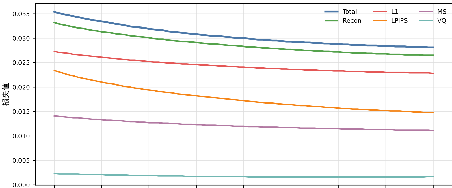
视觉离散表示训练损失曲线
