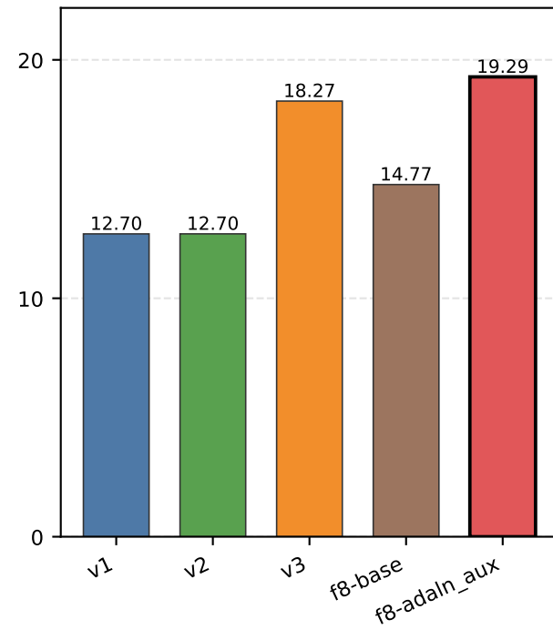
PSNR \uparrow
