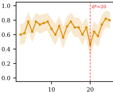
GPT-4o-mini
