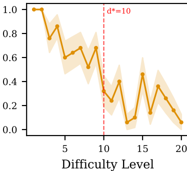
GPT-4o-mini
