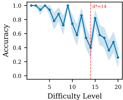
Gemini Flash
