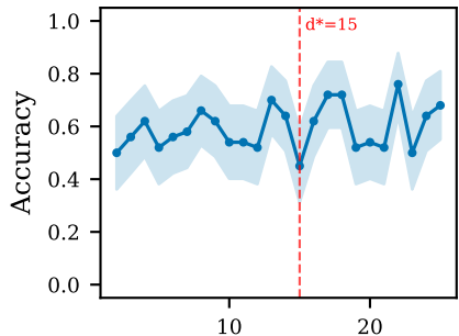
Gemini Flash
